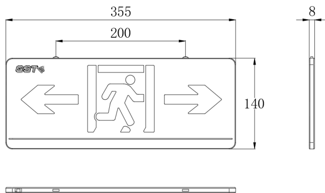
图 1 吊挂式中型双面标志灯具外形示意图（单位：mm）
