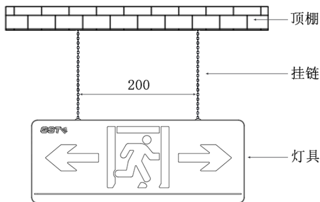
图 1 吊挂式中型双面标志灯具安装示意图（单位：mm）
